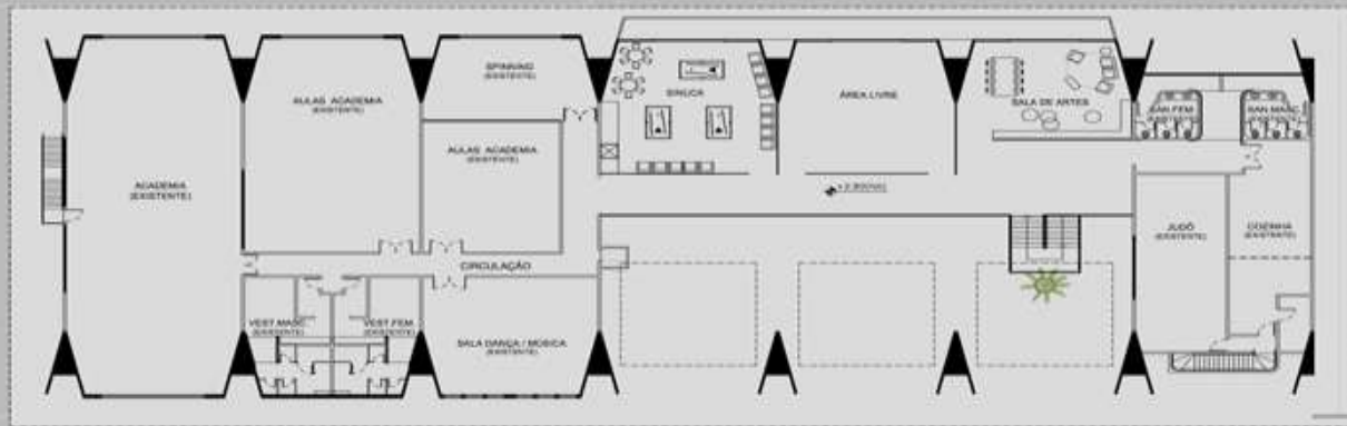
PLANTA PAVIMENTO SUPERIOR / ETAPA 1 - FASE 2 ESQ 1.200
